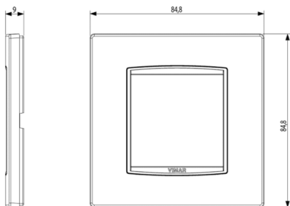
Dessin dimensions hors-tout
